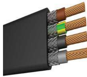
Off-Shore Kabloları
